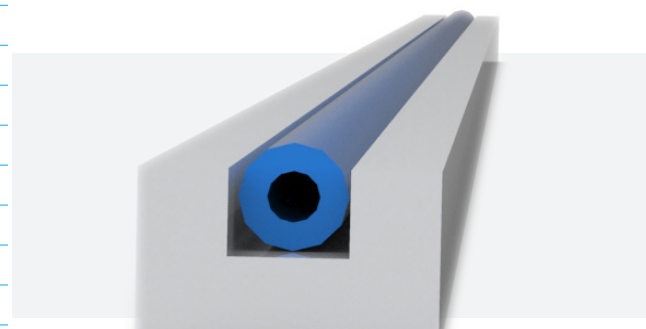
Recommended groove dimensions Machining tolerances : ± 0,05
