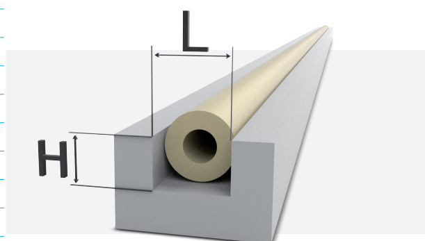
Dimensions recommandées pour la gorge : Tolérance d'usage: ± 0,05
